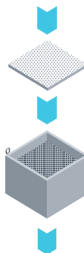
> Feinstaub-Vorfilter M5
